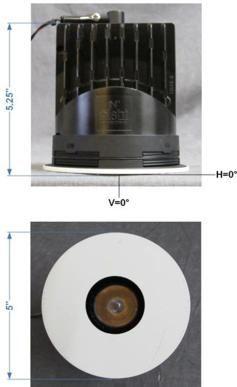
FIG. 1 LUMINAIRE
