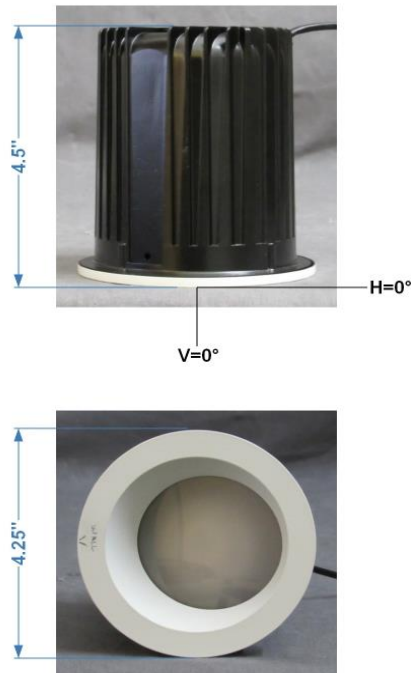
FIG. 1 LUMINAIRE
