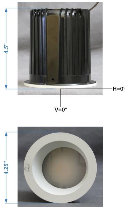
FIG. 1 LUMINAIRE
