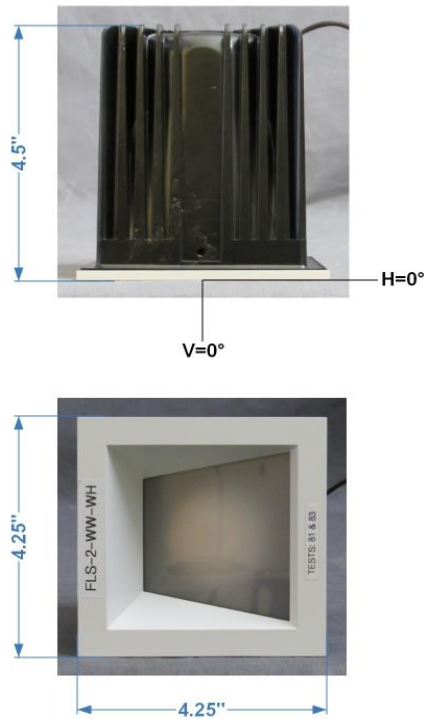
FIG. 1 LUMINAIRE
