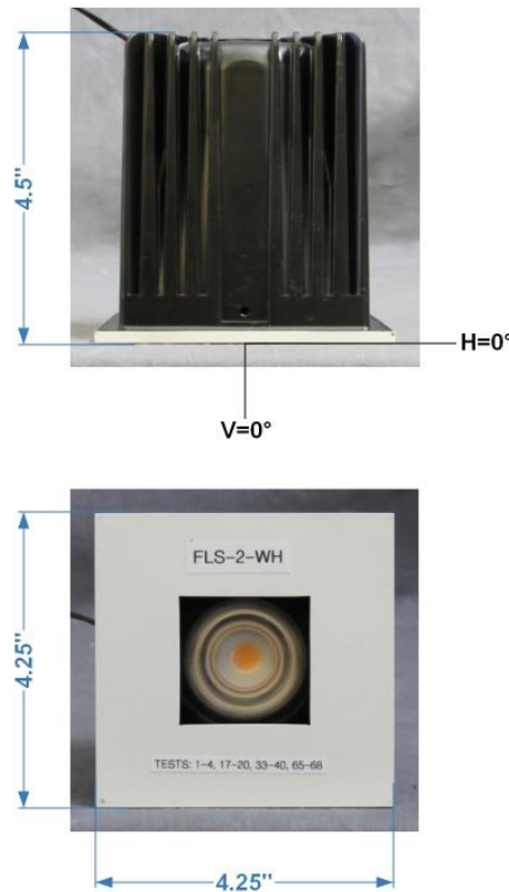
FIG. 1 LUMINAIRE
