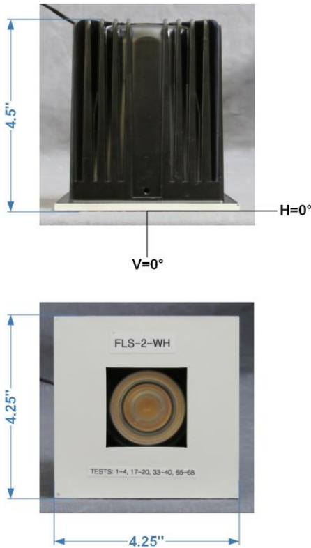
FIG. 1 LUMINAIRE
