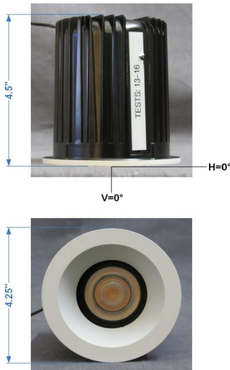
FIG. 1 LUMINAIRE
