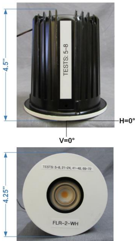
FIG. 1 LUMINAIRE
