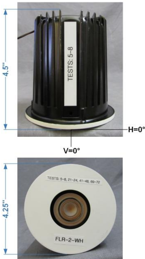
FIG. 1 LUMINAIRE
