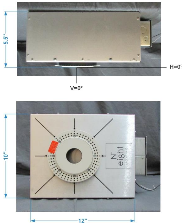
FIG. 1 LUMINAIRE
