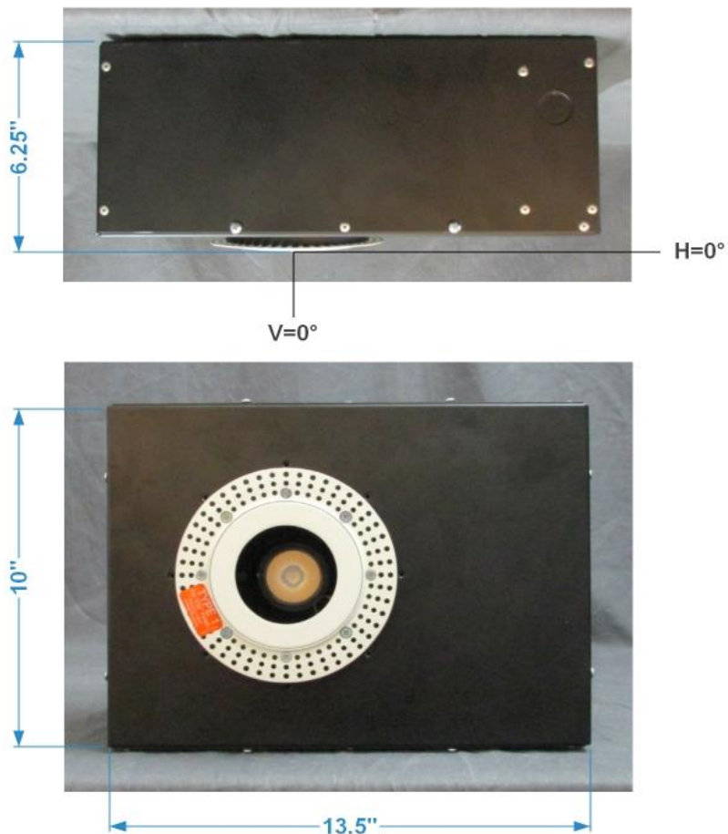
FIG. 1 LUMINAIRE
