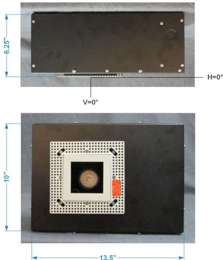
FIG. 1 LUMINAIRE
