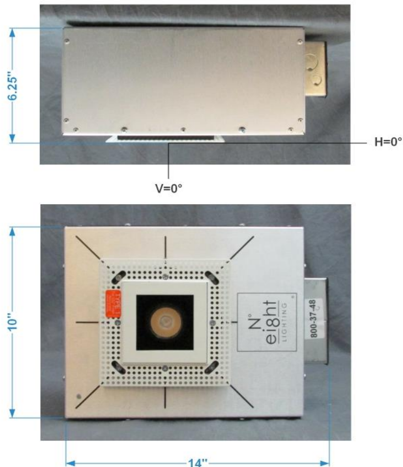
FIG. 1 LUMINAIRE
