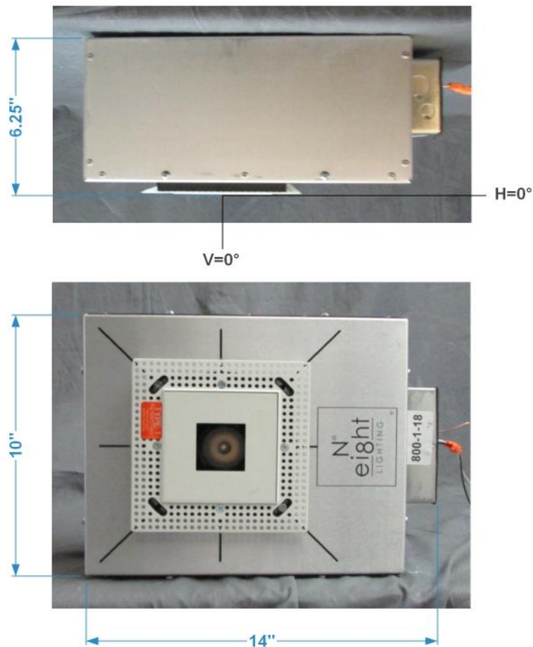
FIG. 1 LUMINAIRE
