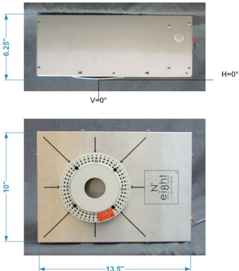
FIG. 1 LUMINAIRE
