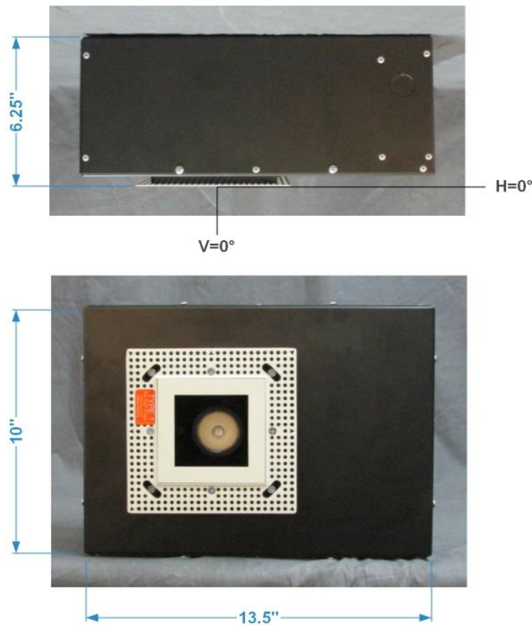
FIG. 1 LUMINAIRE
