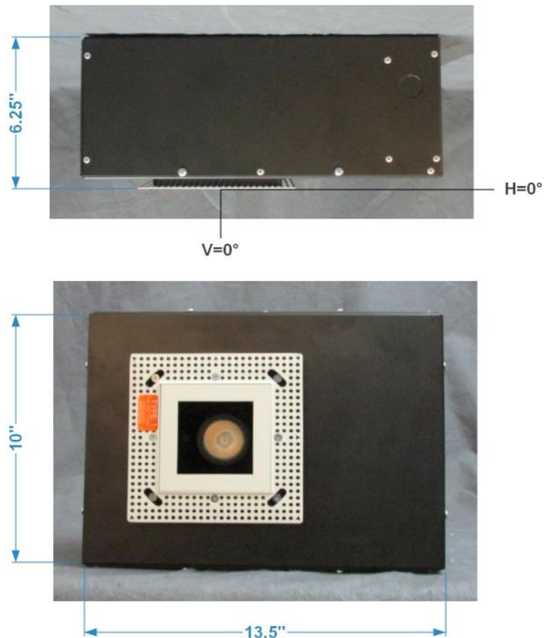
FIG. 1 LUMINAIRE
