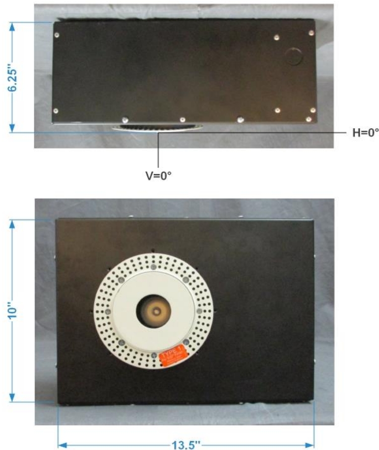
FIG. 1 LUMINAIRE
