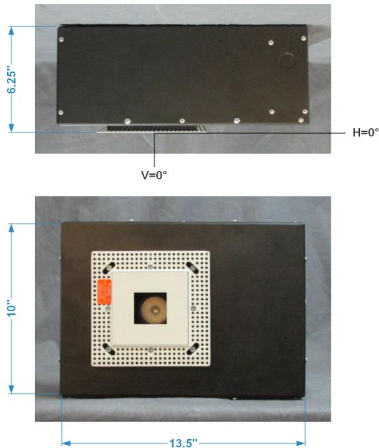
FIG. 1 LUMINAIRE
