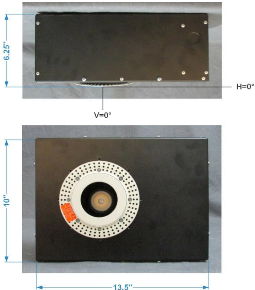
FIG. 1 LUMINAIRE
