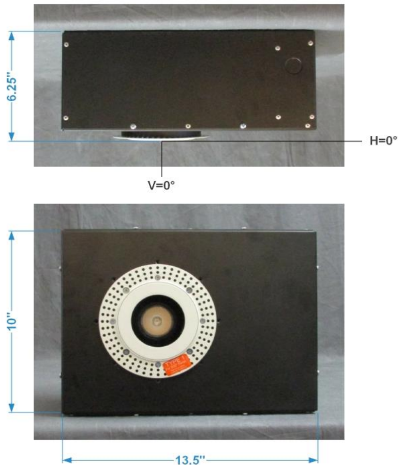
FIG. 1 LUMINAIRE
