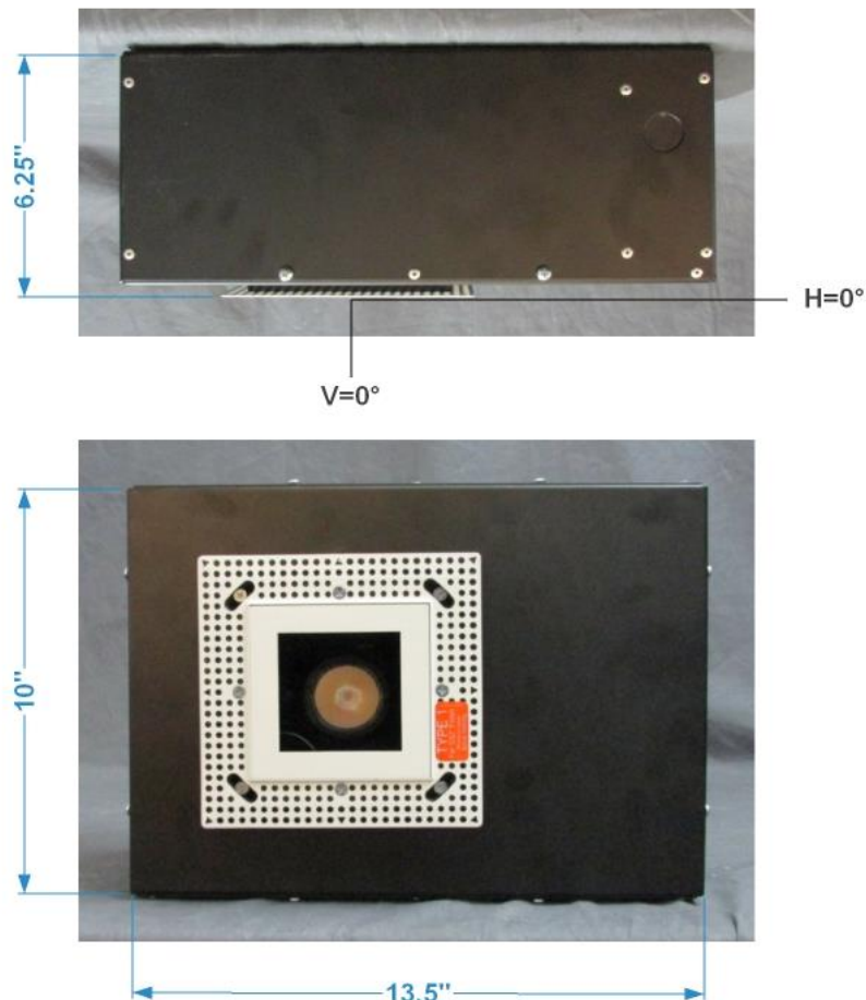
FIG. 1 LUMINAIRE
