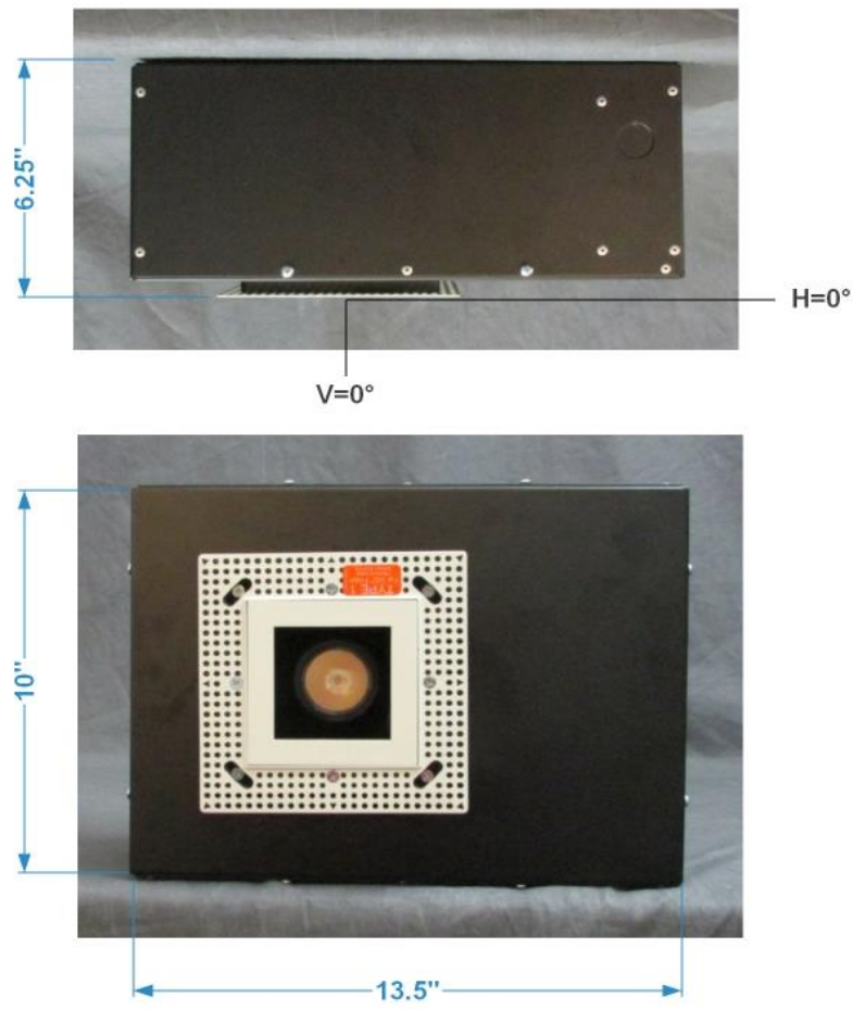
FIG. 1 LUMINAIRE
