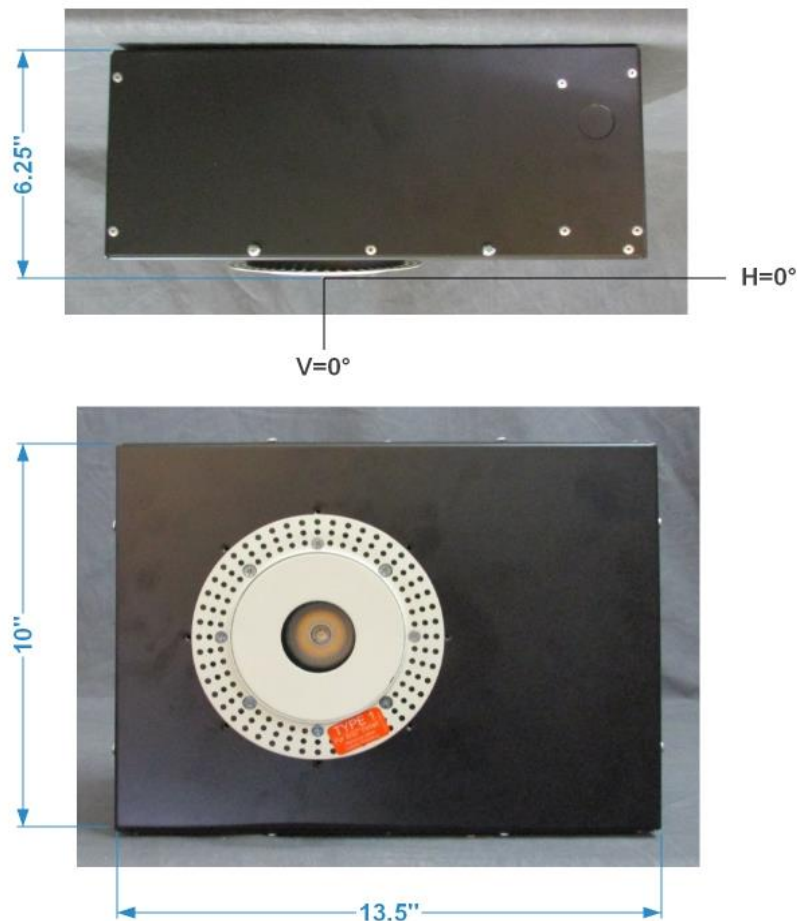
FIG. 1 LUMINAIRE
