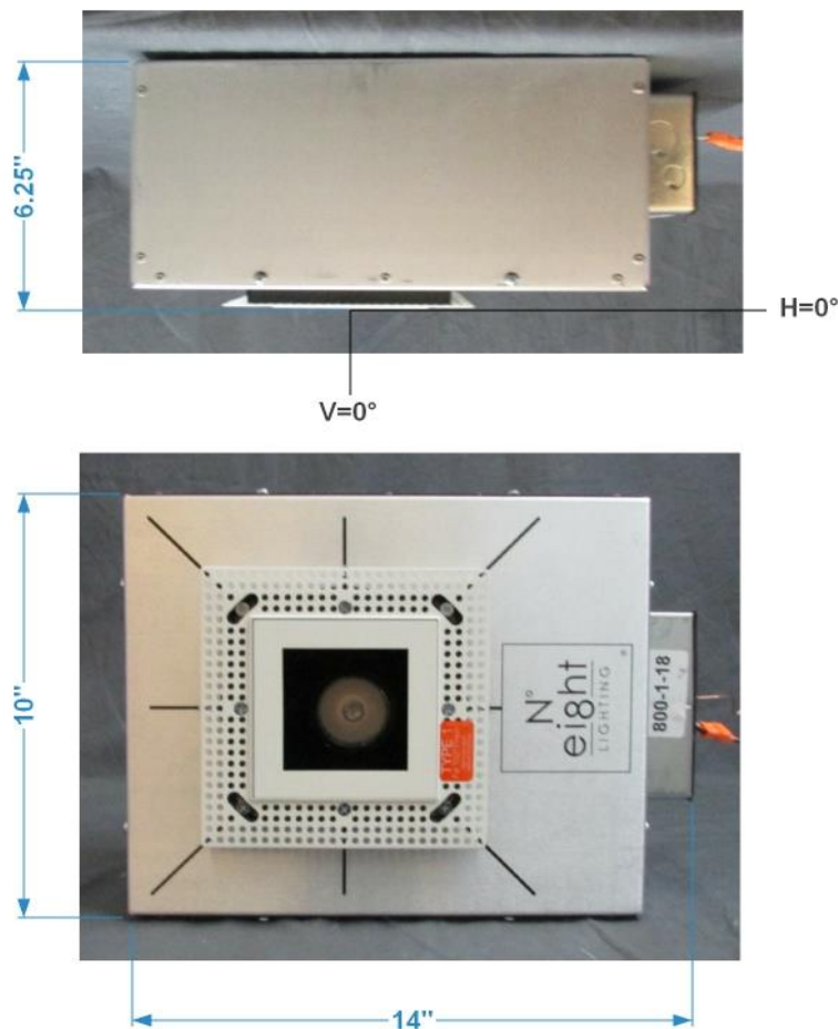
FIG. 1 LUMINAIRE
