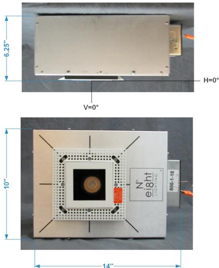
FIG. 1 LUMINAIRE
