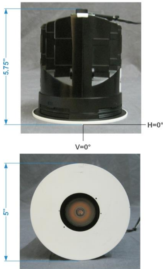
FIG. 1 LUMINAIRE
